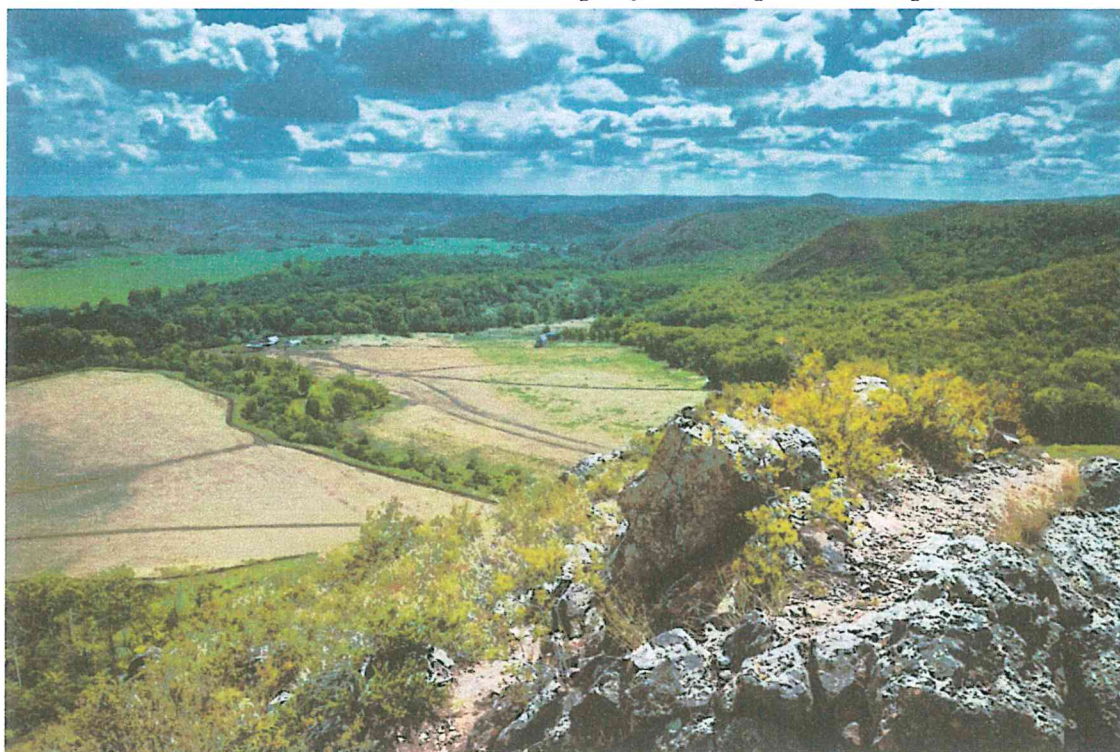
Фото 2. Панорама отрогов хребта Шайтан-Тау с рифовыми известняковыми массивами кембрийского возраста
